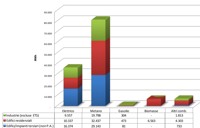
Consumi civili ed industriali [MWh] - Anno 2013
