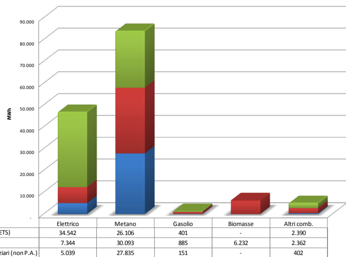
Consumi civili ed industriali [MWh] - Anno 2013
